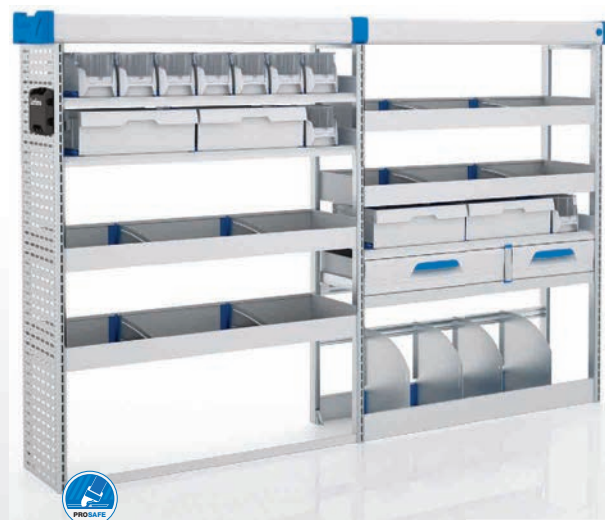
VENSTRE GBLK 11EV Varenr. KR-GBLK11EV Dim. (BxDxH): 2456x382x1530 mm Vægt: 90 kg
