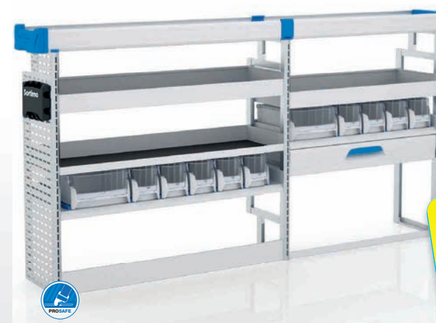
VENSTRE GBLK 7SV Varenr. KR-GBLK7SV Dim. (BxDxH): 2214x382x1196 mm Vægt: 58 kg
